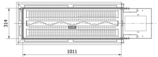
B-B ( 1 : 10 )
