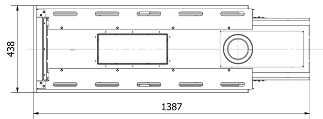
B-B ( 1 : 10 )
